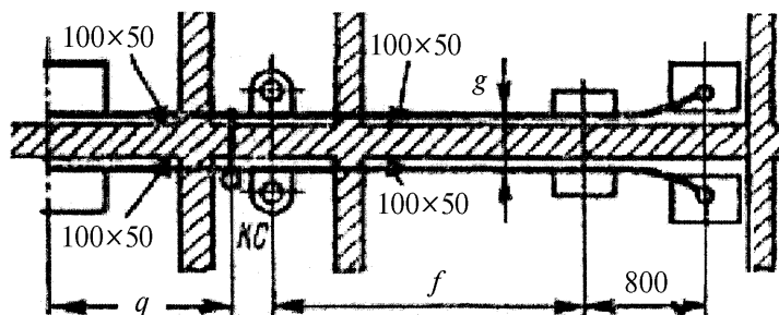
Рисунок 9.1 – Замерно-монтажная карта внутренней канализации
