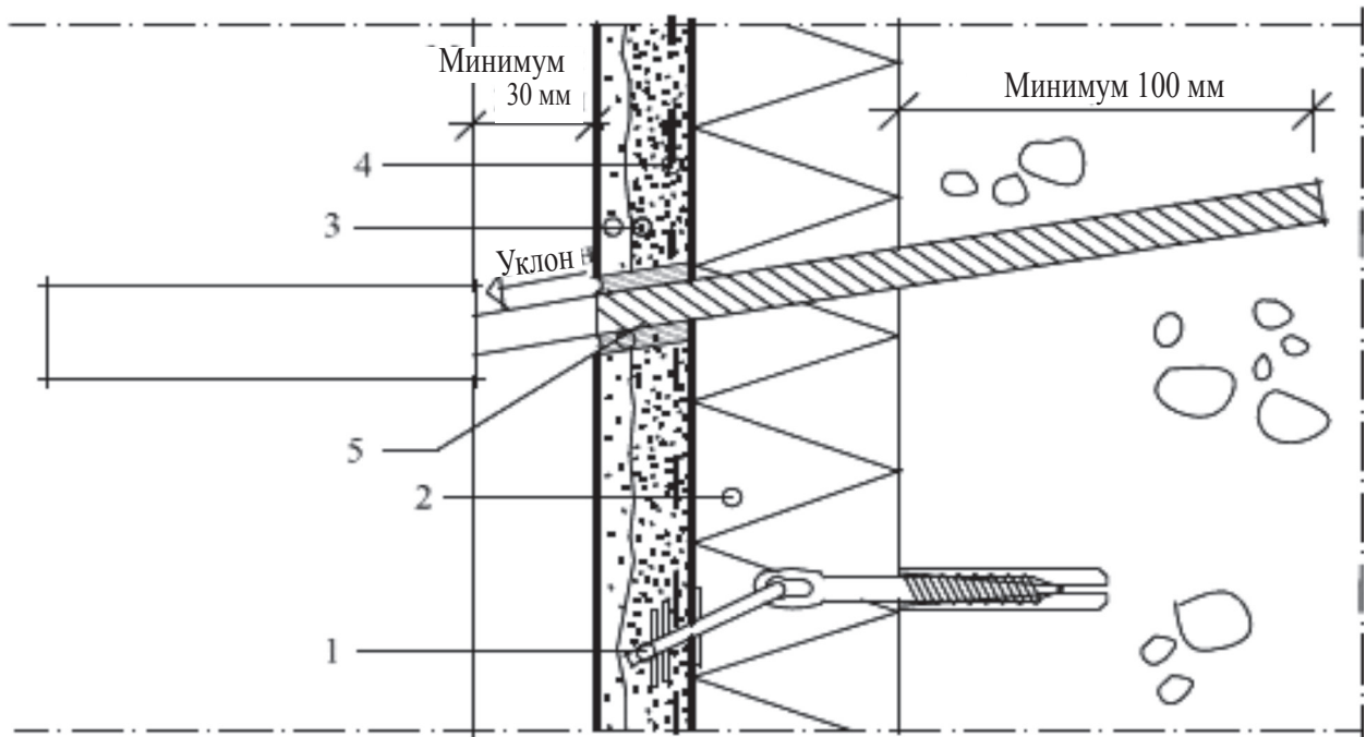
1 – шарнирный анкер; 2 – теплоизоляционный слой; 3 – штукатурный; 4 – армирующая сетка; 5 – эластичная шовная мастика вокруг крепежной детали
