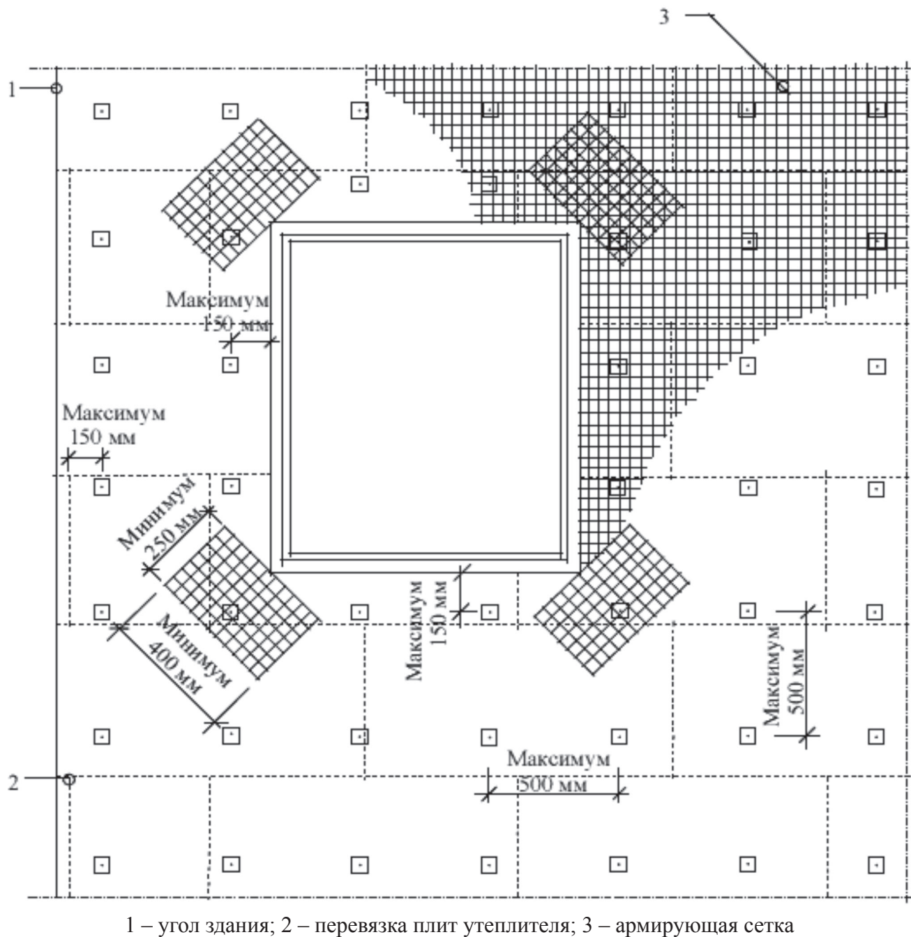
Рисунок 14 – Усиление вершин углов проемов в основании
