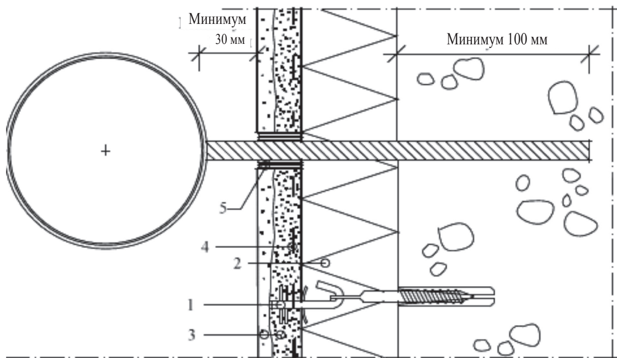
1 – шарнирный анкер; 2 – теплоизоляционный слой; 3 – штукатурный слой; 4 – армирующая сетка; 5 – эластичная шовная мастика вокруг крепежной детали
