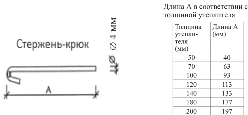
Рисунок 7 – Стержень-крюк шарнирного анкера
