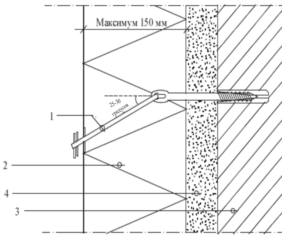
1 – шарнирный анкер; 2 – теплоизоляционный слой; 3 – основание
