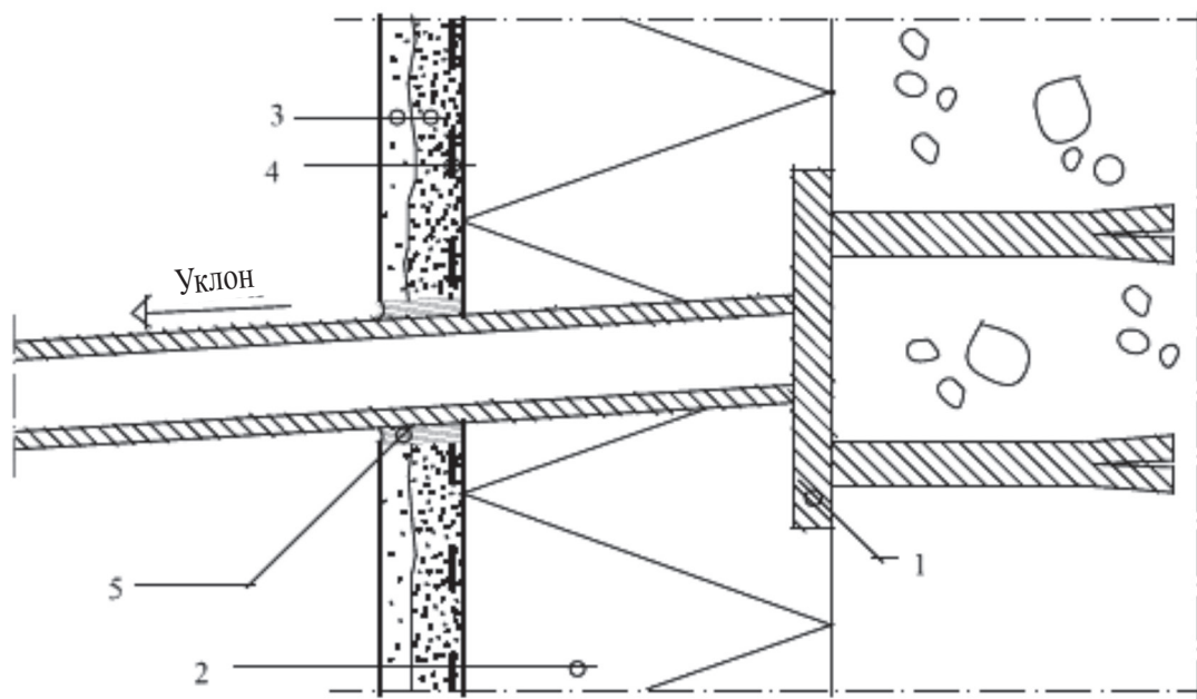
Рисунок 9.8 – Устройство системы в месте устройства воздухопроводов
