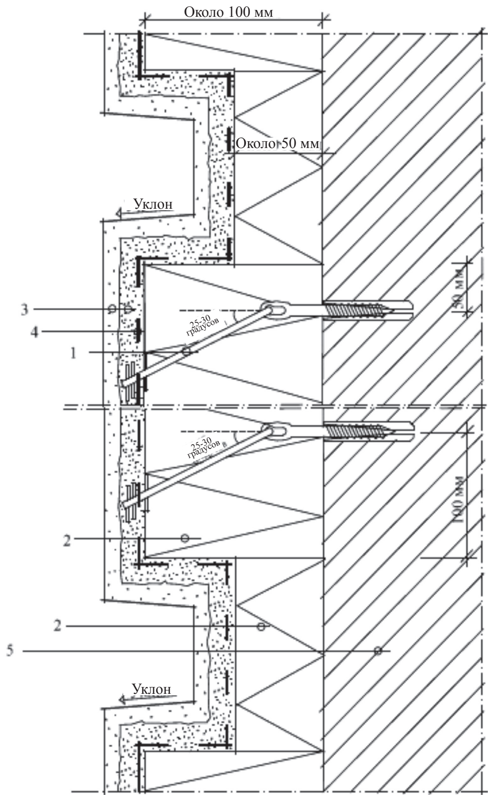
1 – шарнирный анкер; 2 – теплоизоляционный слой; 3 – штукатурный слой; 4 – армирующая сетка; 5 – наружная стена
