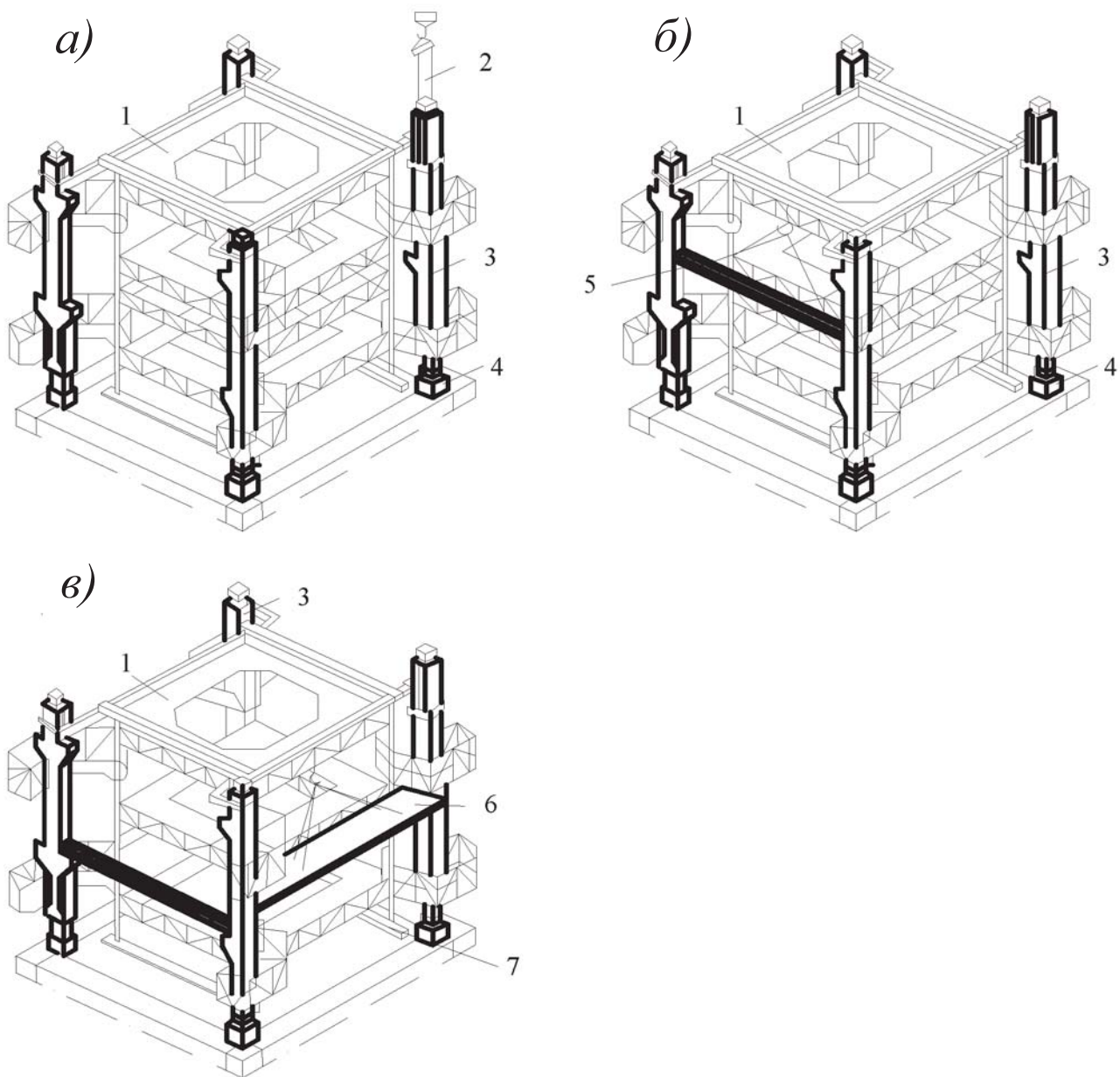
а) установка колонн; б) укладка ригелей нижнего этажа; в) укладка плит нижнего этажа 1 – РШИ; 2 – траверса; 3 – колонна; 4 – оголовок нижестоящей колонны; 5 – ригель; 6 – плита; 7 – подкладочный брус
