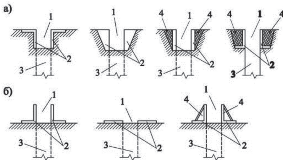
а) заглубленная форшахта; б) наземная форшахта
