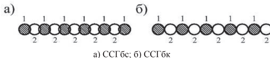
1, 2 – последовательность устройства свай Рисунок 2 – Типовые схемы устройства ССГ
