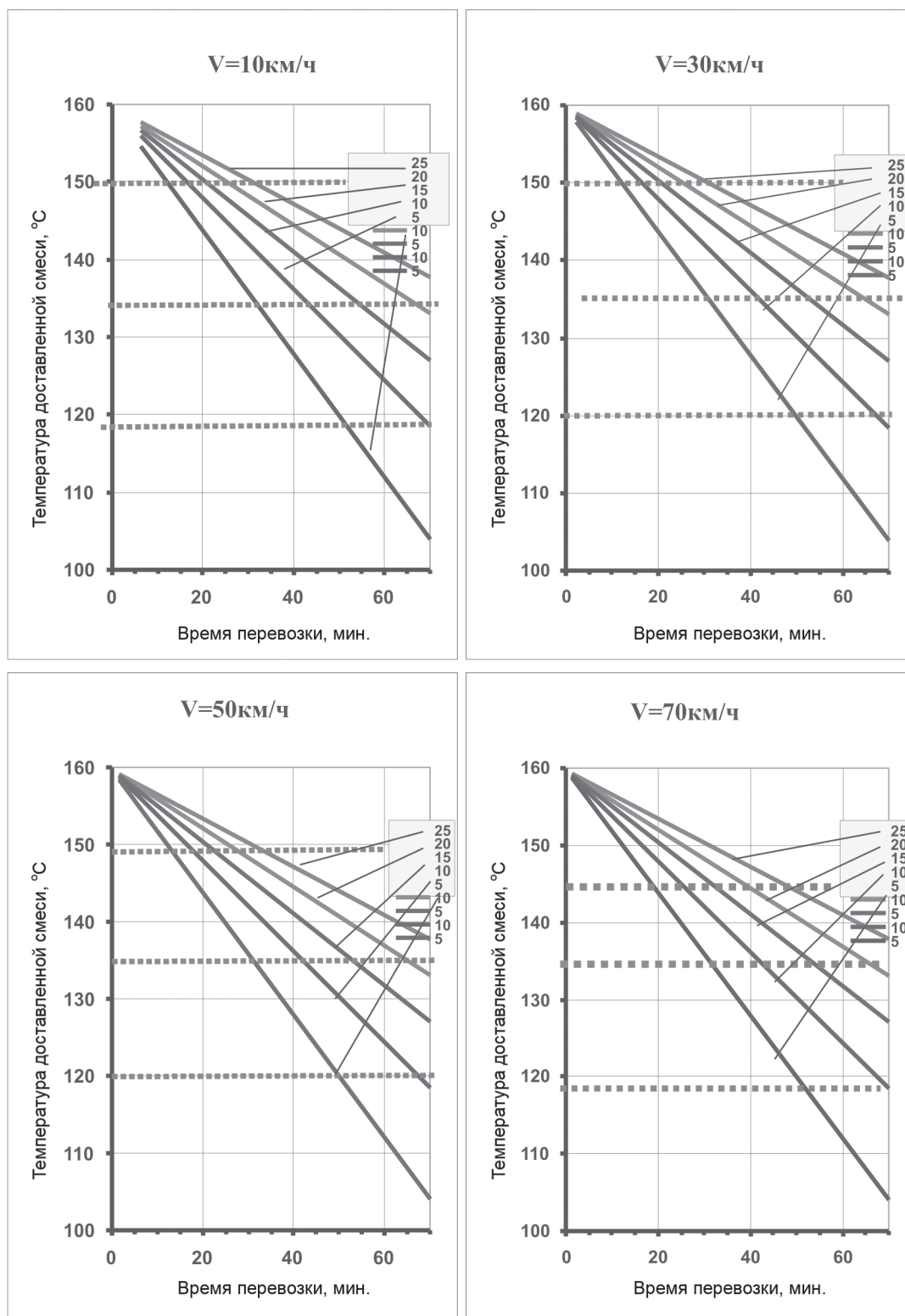
Рисунок Д.1 – Время перевозки горячей асфальтобетонной смеси в автомобилях-самосвалах при температуре отгрузки t_{нач} = 160 \text{ } ^\circ\text{C} (цифры на лучах – температура воздуха)
